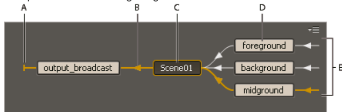
A. Marker, der anzeigt, dass die Komposition nicht in andere Kompositionen fließt B. Flussrichtung C. Aktive (aktuelle) Komposition D. Upstream-Kompositionen E. Marker, die anzeigen, dass andere Kompositionen in diese Kompositionen fließen
