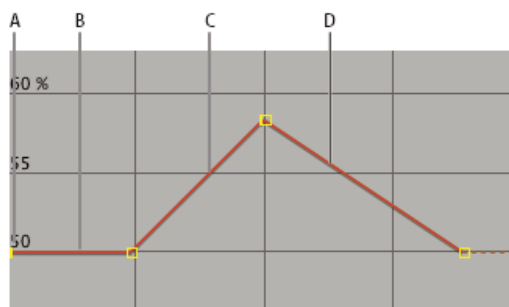
Wertkurve
