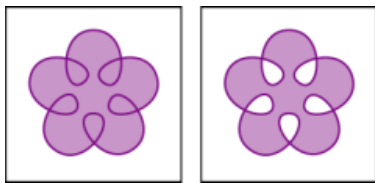
Sich selbst schneidender Pfad mit der Füllregel Nicht-Null (links) im Vergleich mit der Füllregel Gerade-Ungerade (rechts)
