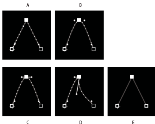
Bewegungspfad-Interpolation
