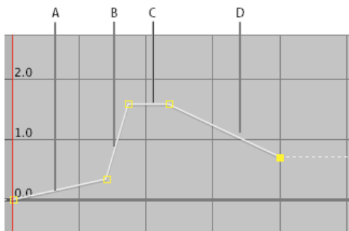
Zeitverzerrungskurve
